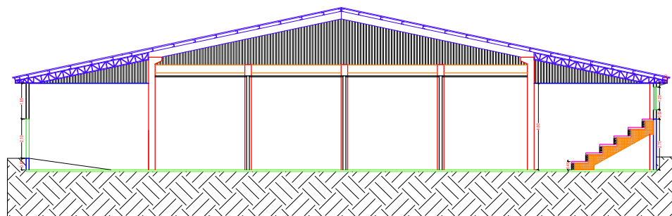
Corte AA
